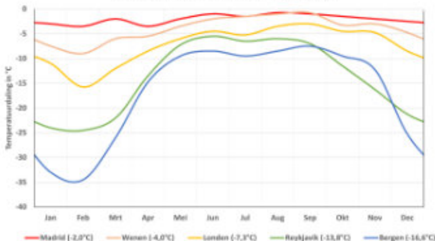
Temperatuurdaling t.o.v. heden in 100 jaar
